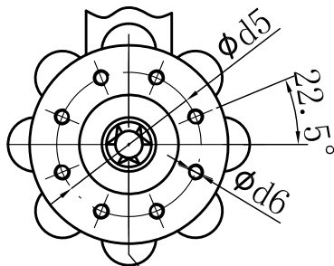
BA1~BA4法兰 A向
