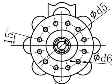
BA5法兰 A向
